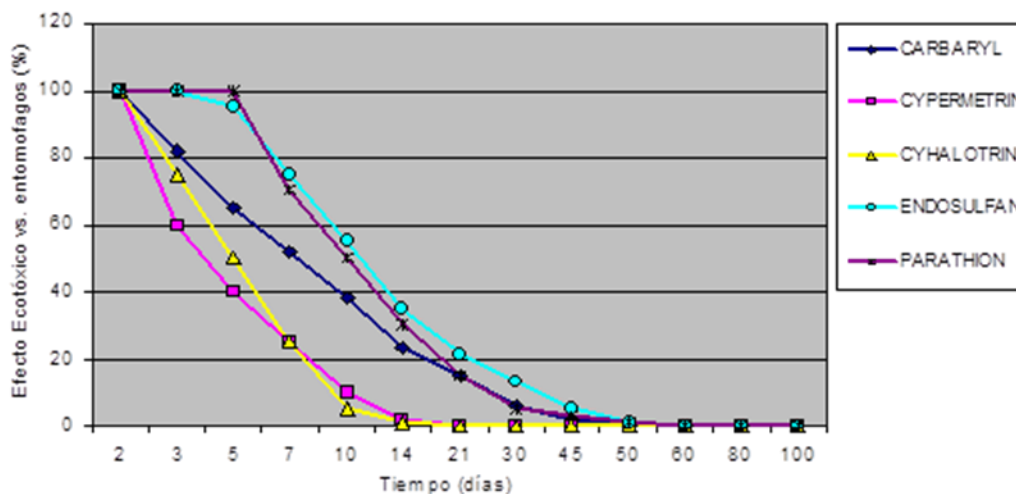
Figura 4.- Curvas de efecto vs tiempo de insecticidas en suelo.
